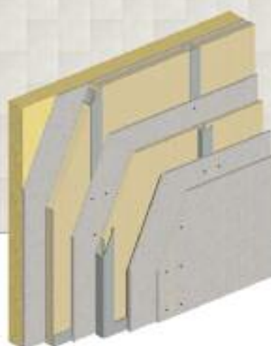
Parete con finitura esterna a cappotto
