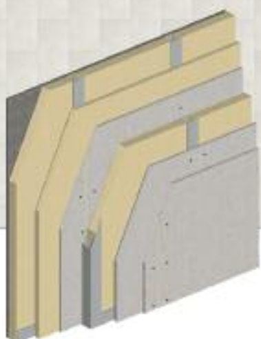
Parete con finitura esterna in lastre cementizie FERMACELL Powerpanel H 2 O
